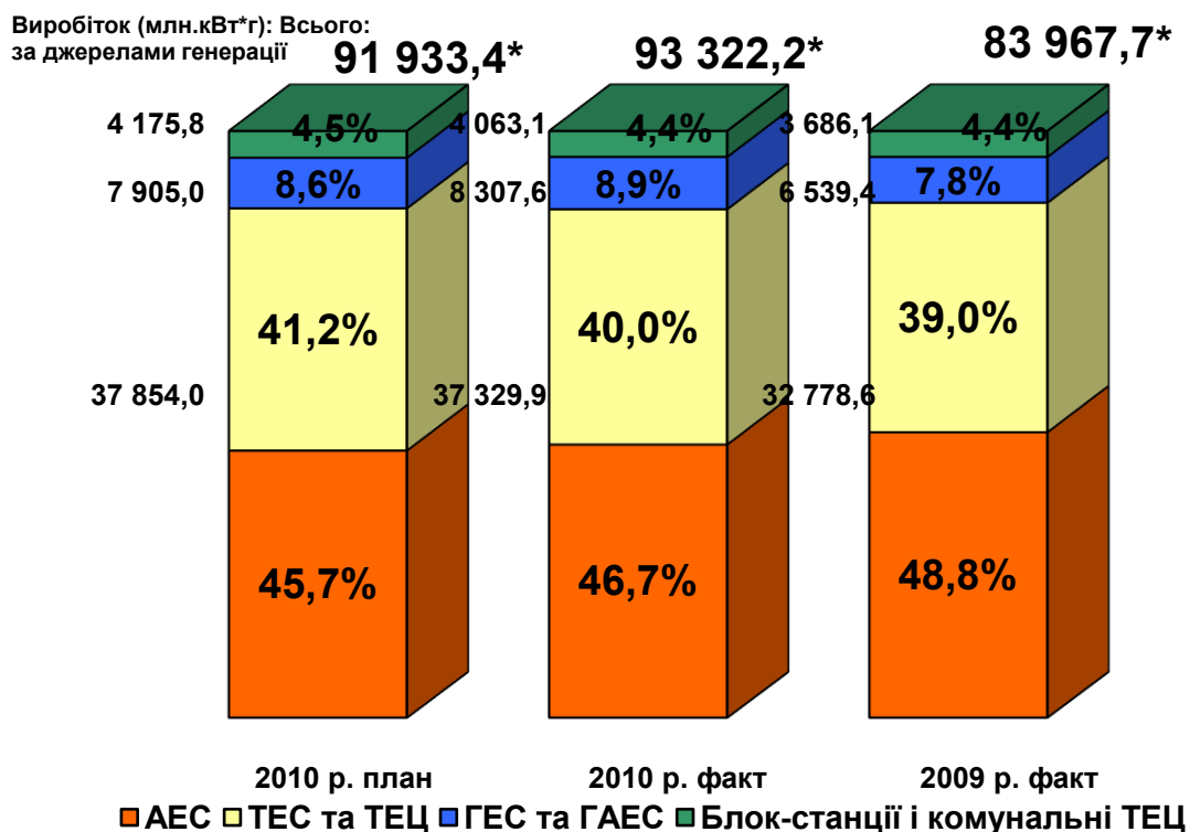
Структура та обсяги виробництва електроенергії по ОЕС України за 6 місяців 2009, 2010 рр.
