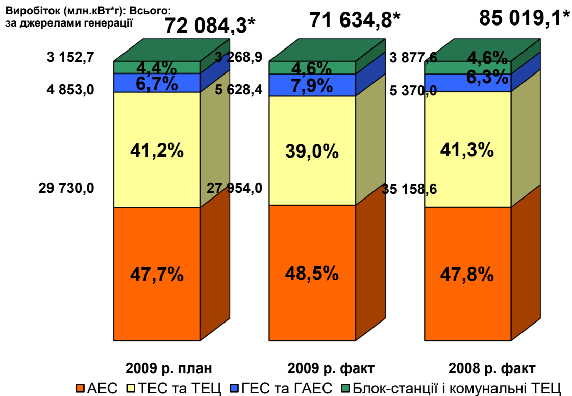
Структура та обсяги виробництва електроенергії по ОЕС України за 5 місяців 2008 - 2009 рр.
