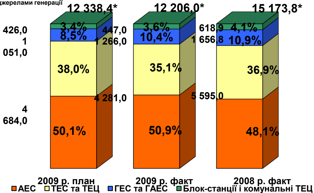
Структура та обсяги виробництва електроенергії по ОЕС України у травні 2008, 2009 рр., млн.кВт·г
