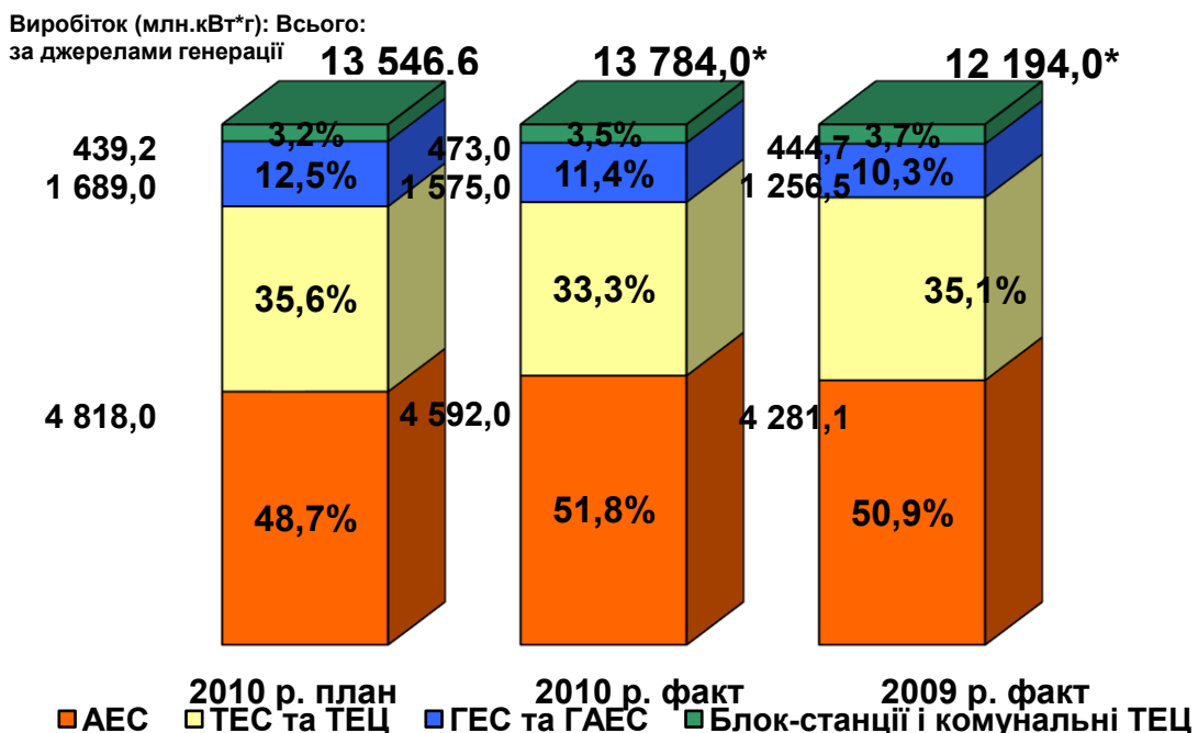
Структура та обсяги виробництва електроенергії по ОЕС України у травні 2009, 2010 рр., млн.кВт·г
