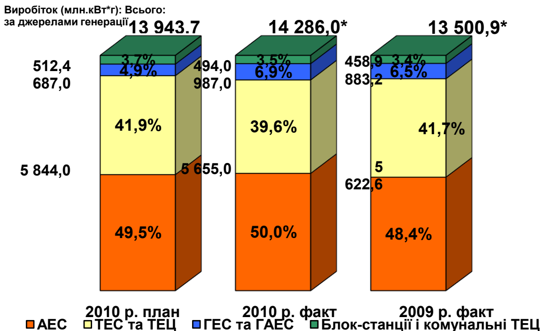
Структура та обсяги виробництва електроенергії по ОЕС України у липні 2009, 2010 рр., млн.кВт·г
