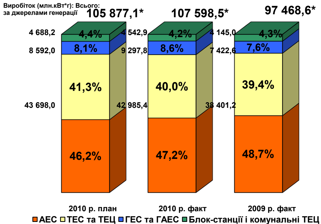
Структура та обсяги виробництва електроенергії по ОЕС України за 7 місяців 2009, 2010 рр.
