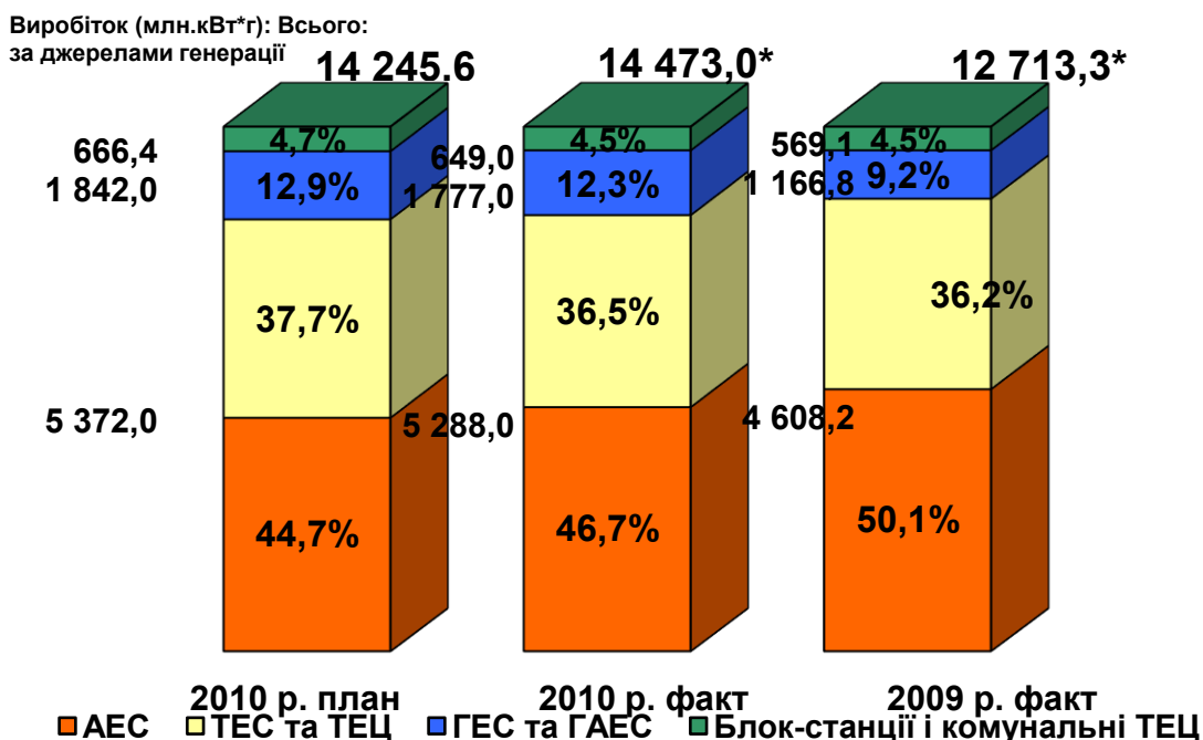
Структура та обсяги виробництва електроенергії по ОЕС України у квітні 2009, 2010 рр., млн.кВт·г
