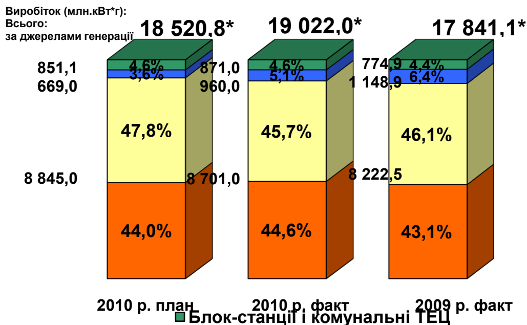
Структура та обсяги виробництва електроенергії по ОЕС України у грудні 2009, 2010 рр., млн.кВт·г
